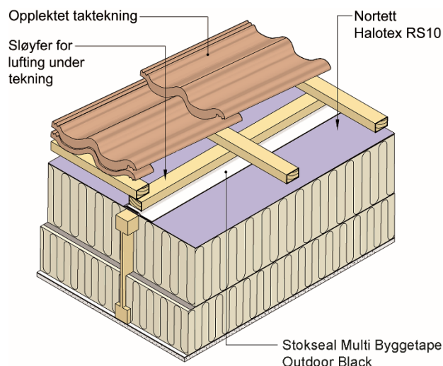
Fig. 1 Stokseal Multi Byggtape Outdoor Black brukt på omleggsskjøter av Nortett Halotex RS10 undertak
