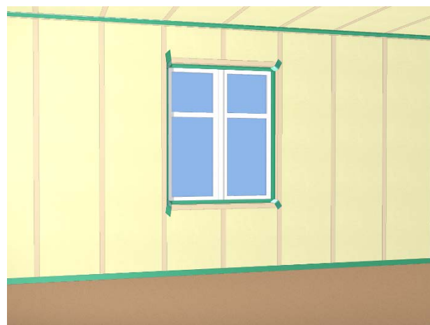
Fig. 2 Stokseal Multi Byggtape brukt til forsegling av skjøter i dampsperrersjiktet.
