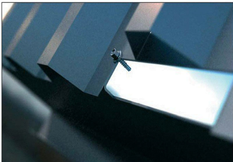
Montage av stålplatta på stålprofil
